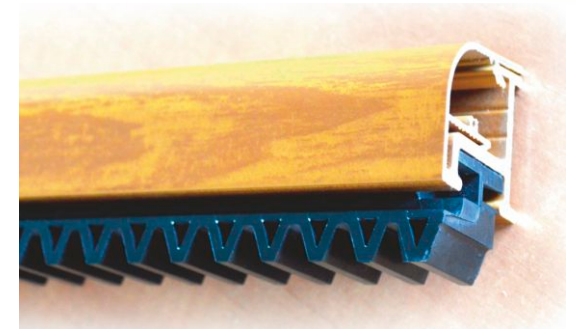
CACHE CRÉMAILLÈRE EN ALUMINIUM ET CRÉMAILLÈRE EN NYLON
