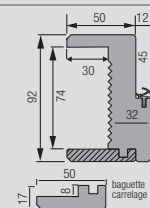
KM1 cloison 72 mm rive droite
